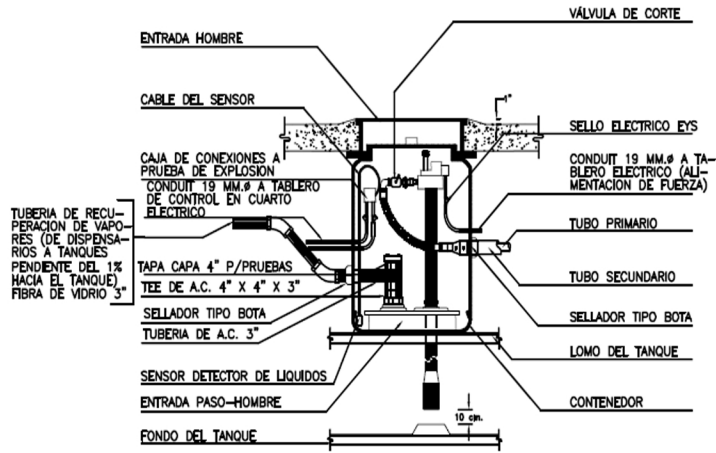
CORTE ESQUEMÁTICO SIN ESCALA ACOT.: CMS.
