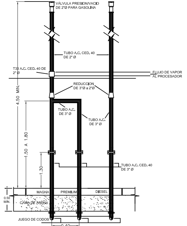
CORTE ESQUEMATICO SIN ESCALA ACOT.: CMS.
